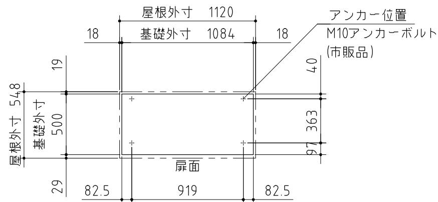
ベタ基礎図
