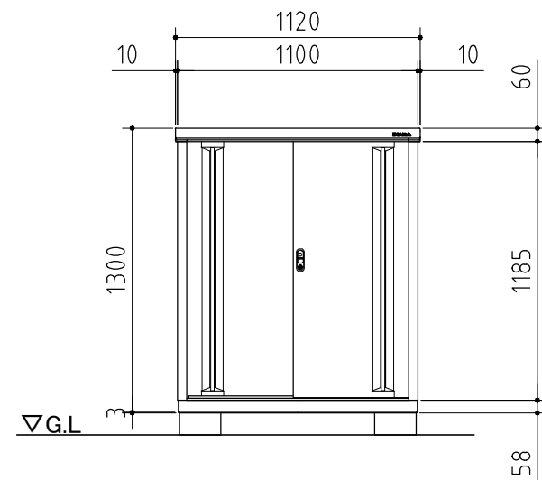
正面図
